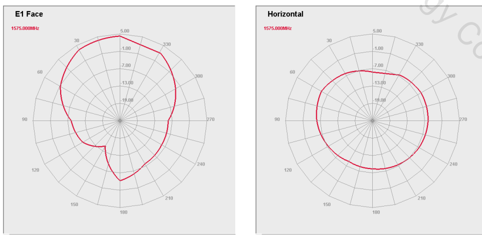
E-Plane
