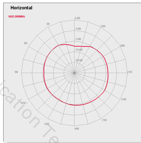
H-Plane
